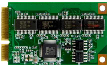
图二： TPM-4COM VER:1.0 产品背面图
