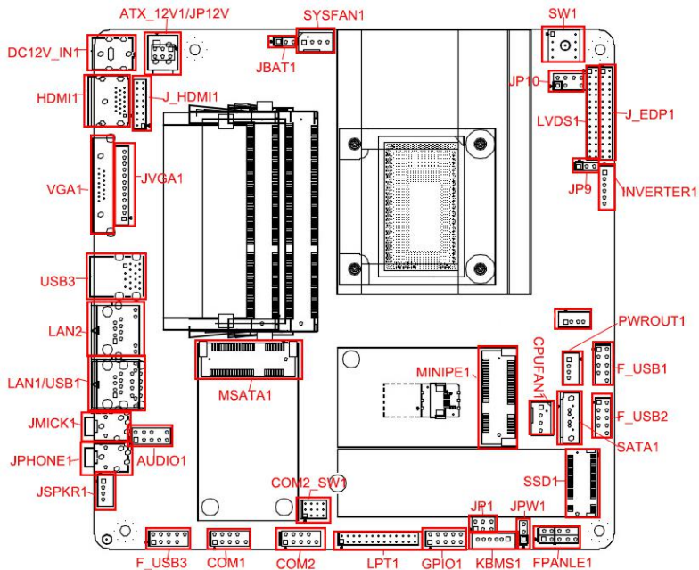
ITX-B671 接口位置图
