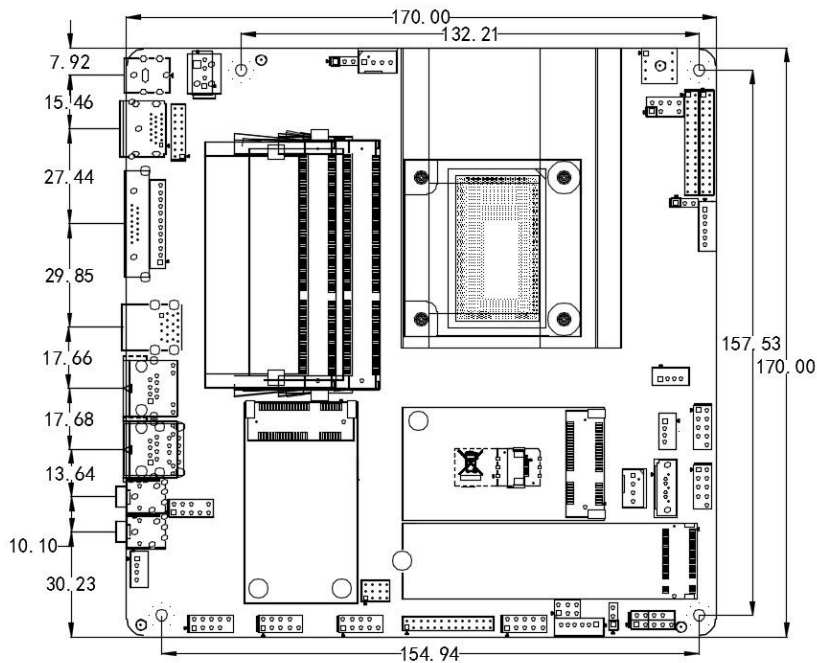
ITX-B671 VER:1.1尺寸图
