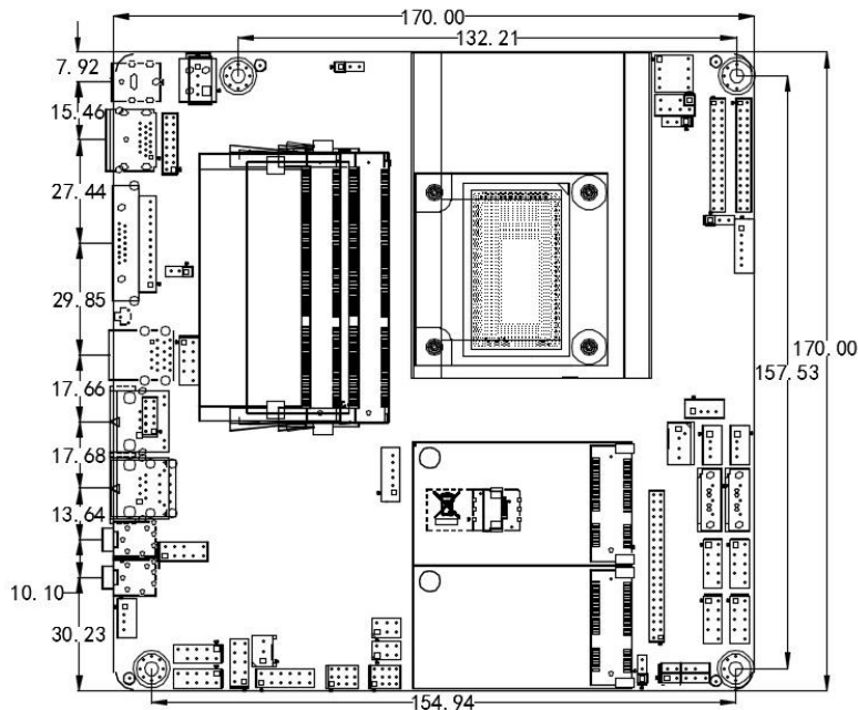
ITX-B670 VER:1.3A尺寸图
