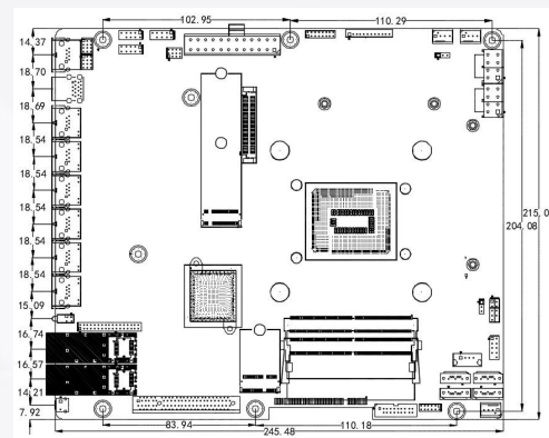
产品尺寸图：
