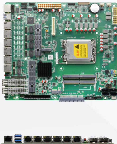
接口标示图：
