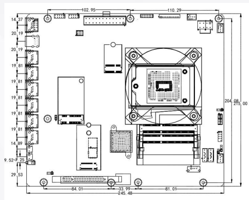
产品尺寸图：
