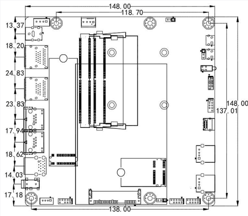
产品尺寸图：
