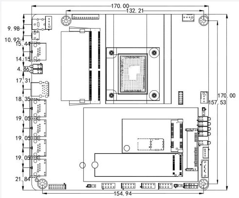
产品尺寸图：
