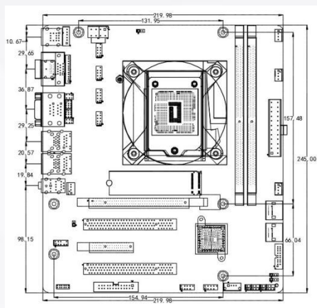
产品尺寸图:
