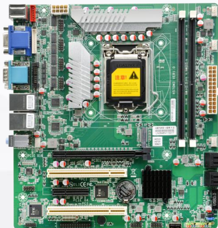
接口标示图：
