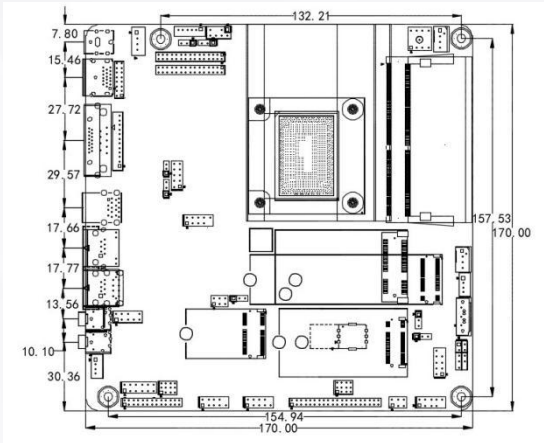
产品尺寸图：
