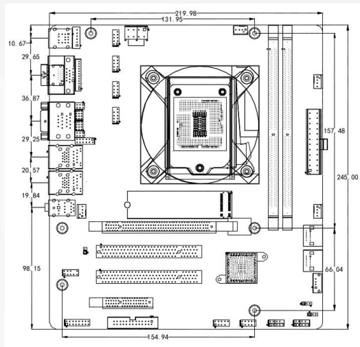
产品尺寸图：
