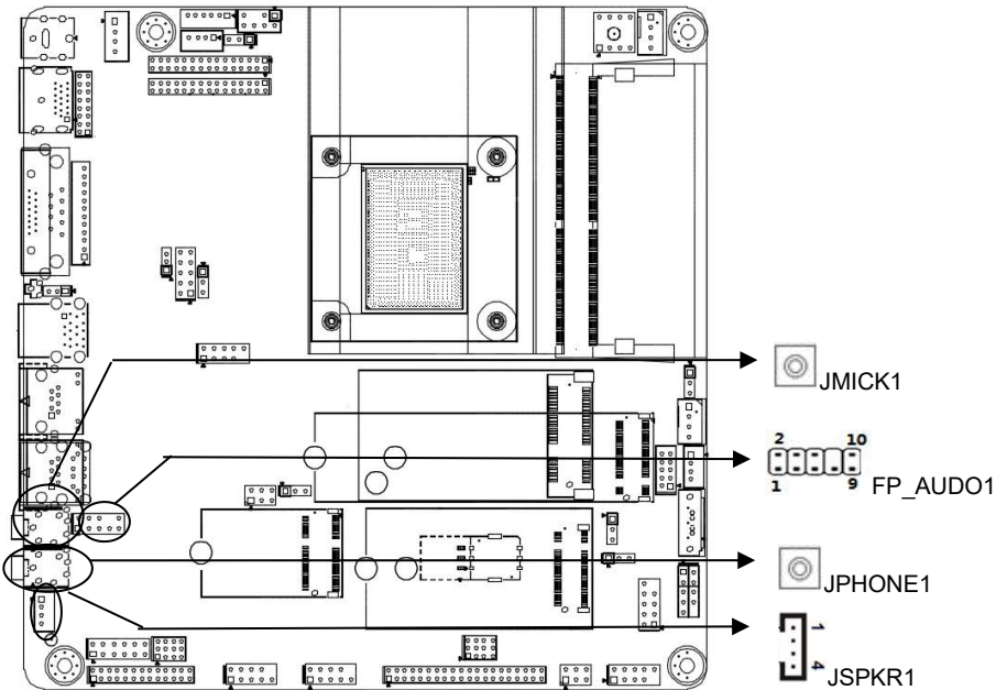
FP_AUDIO1（前置音频）定义:
