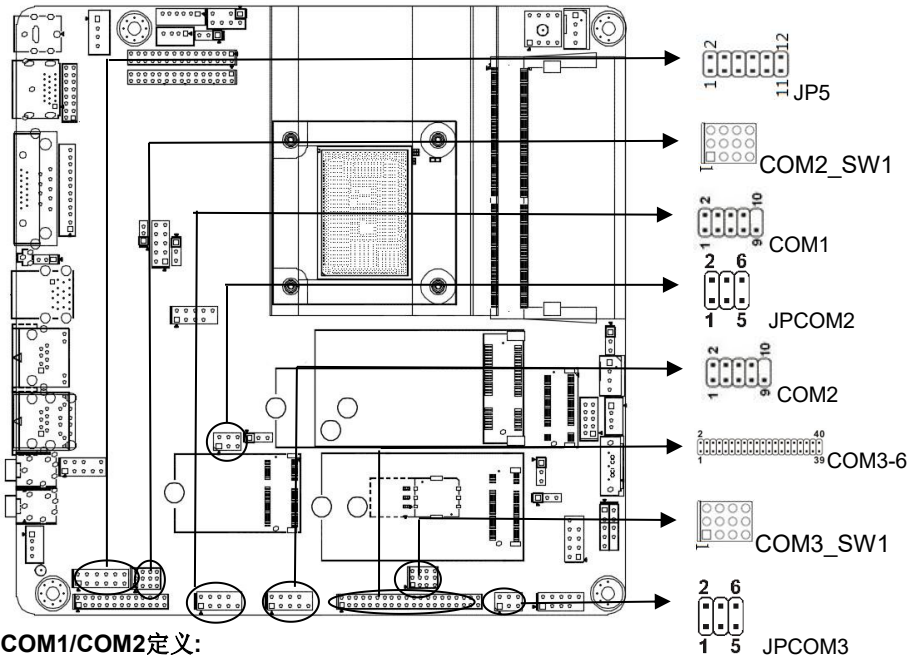
COM1/COM2定义:
