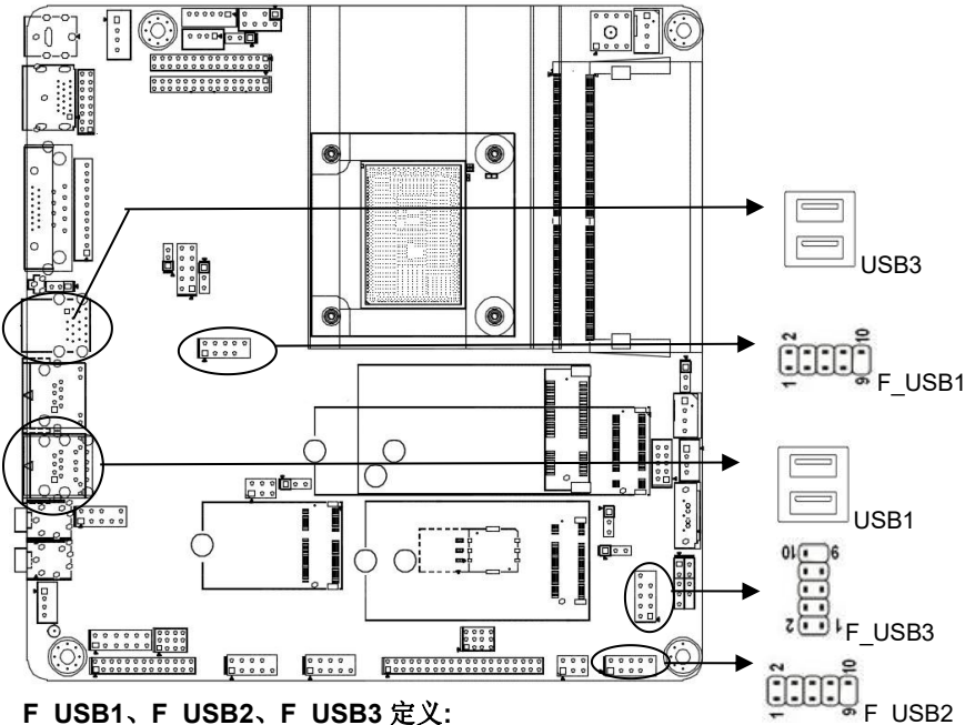
F_USB1、F_USB2、F_USB3 定义:
