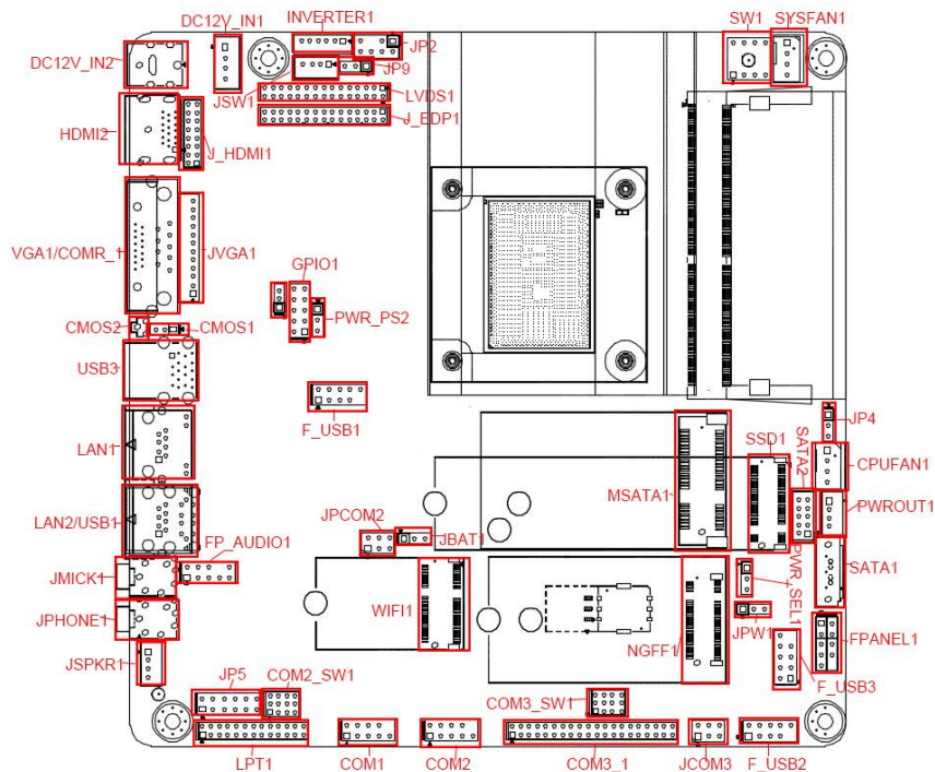
ITX-B641 VER:1.1A 接口位置图
