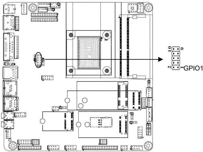
GPIO1 定义:
