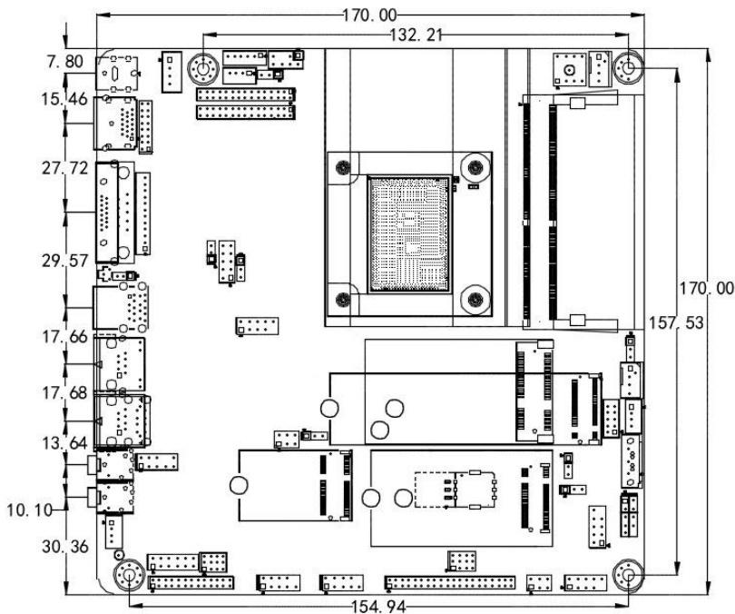
ITX-B641 VER:1.1A 尺寸图
