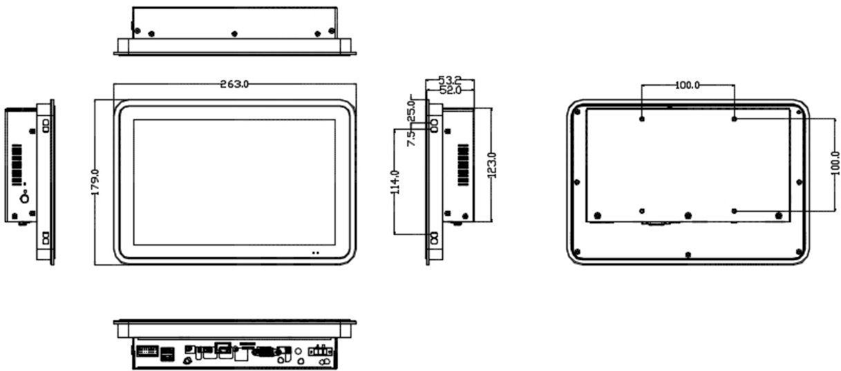
尺寸图
