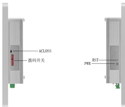
侧面 I/O 视图
