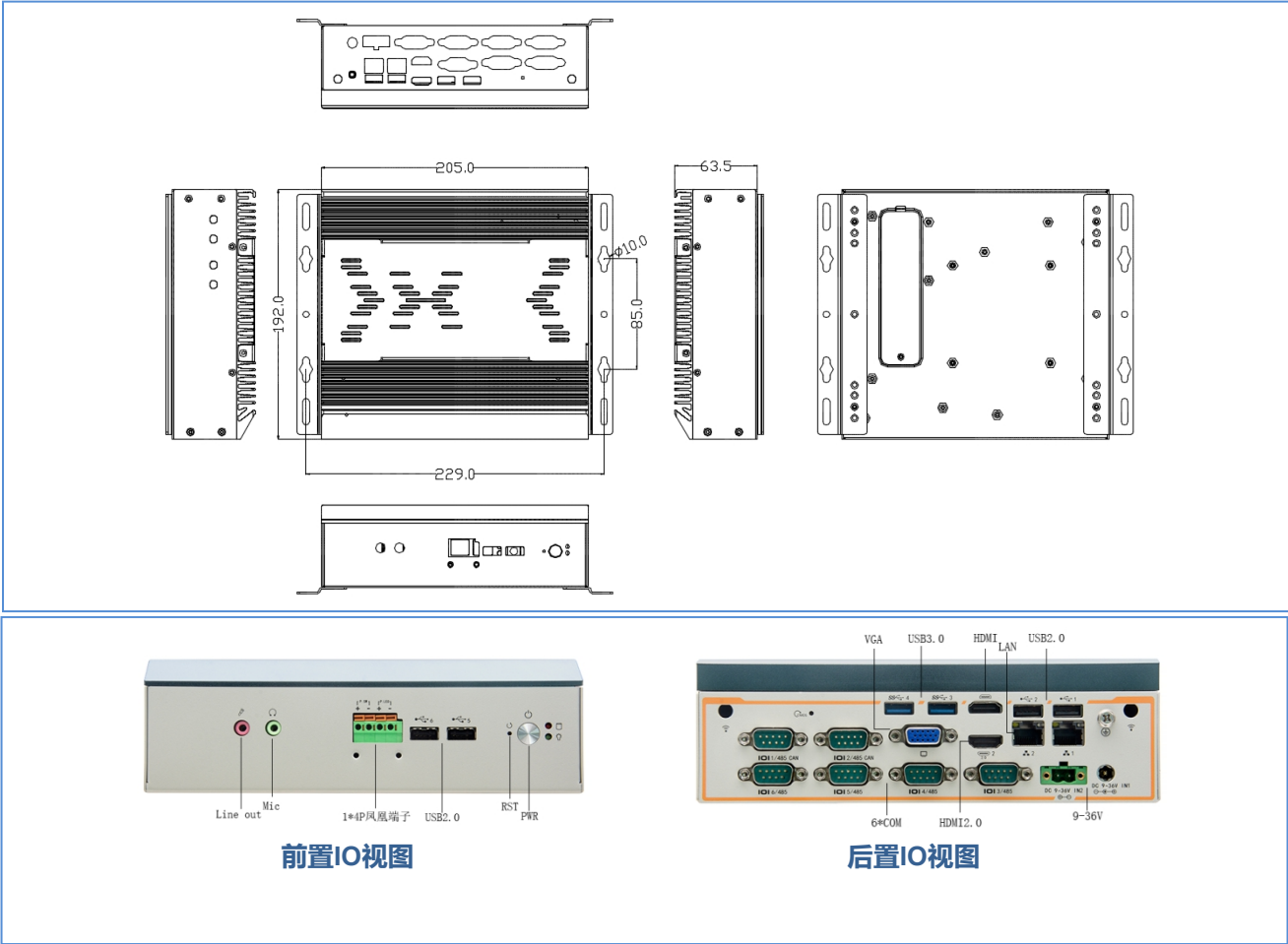
尺寸图
