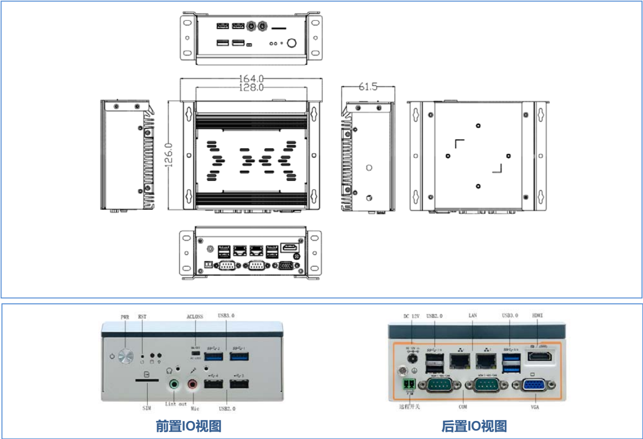
尺寸图
