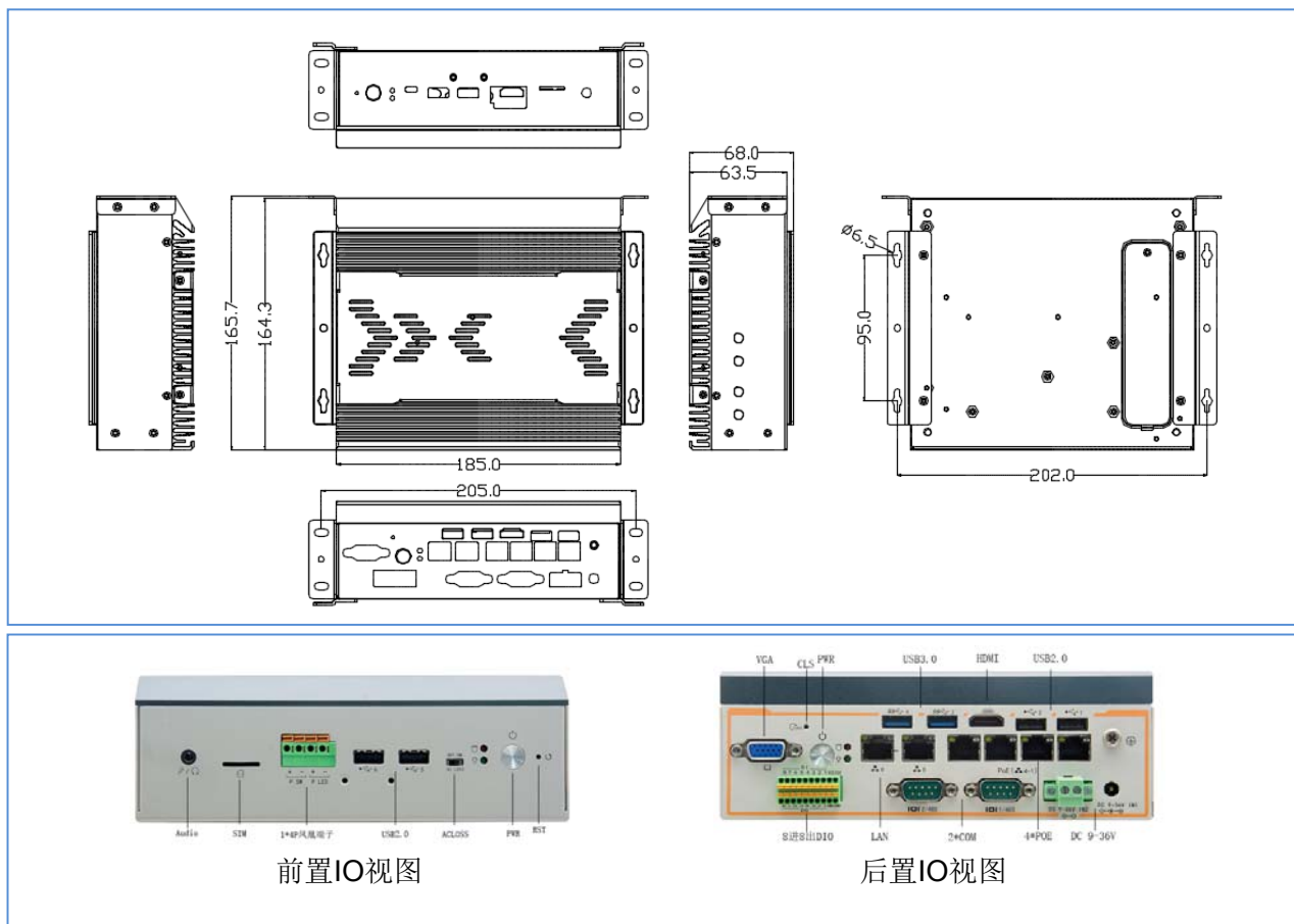
尺寸图
