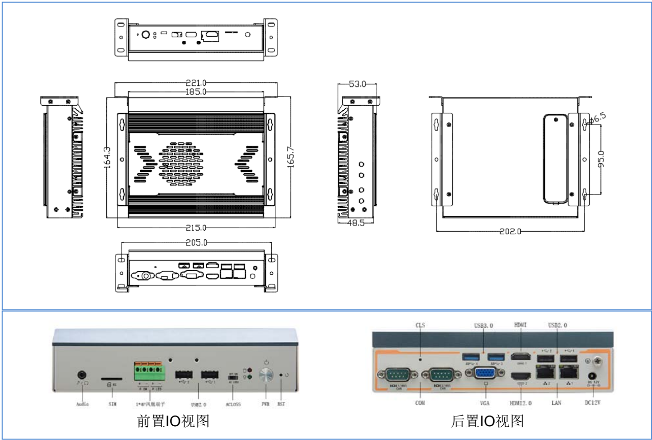
尺寸图
