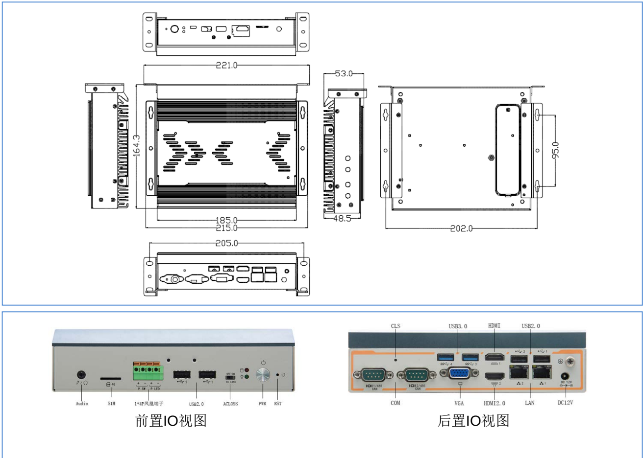
尺寸图
