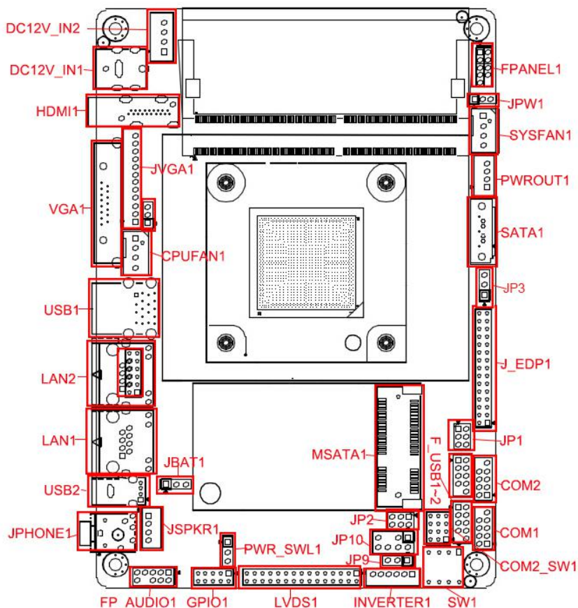
EPIC-E42 接口位置图
