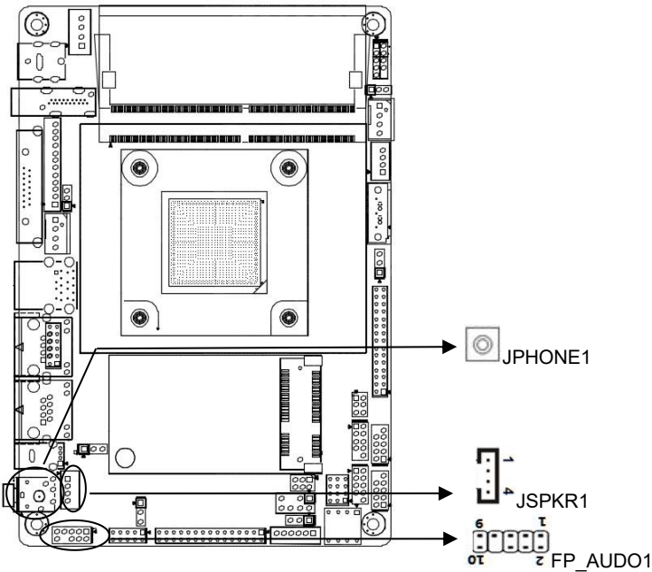
FP_AUDIO1（前置音频）定义:
