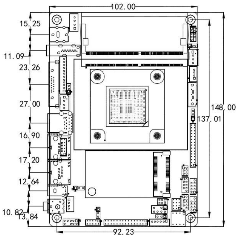
EPIC-E42 VER:1.0 尺寸图
