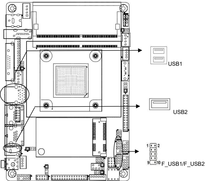
F_USB1、F_USB2 定义:
