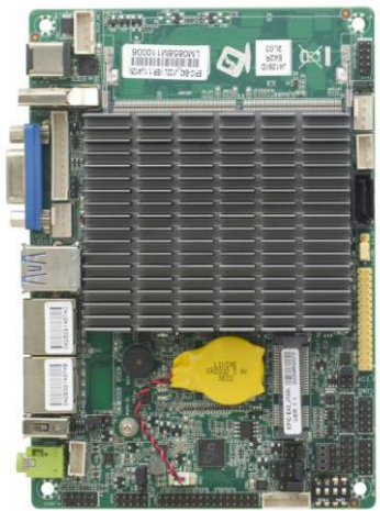
图一：EPIC-E42 VER:1.1 主板正面图
