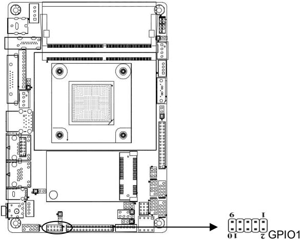
GPIO1 定义:
