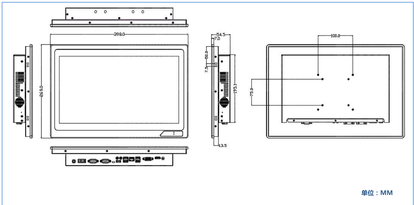
前面板视图
