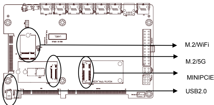
(M211-IO 示意图)
