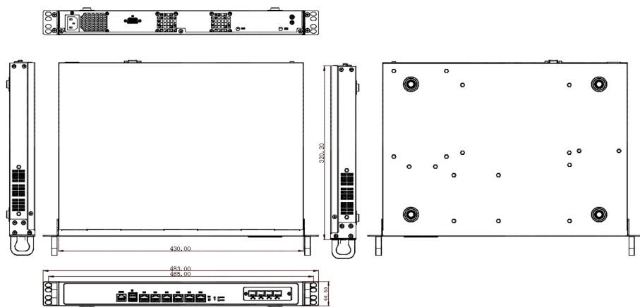
R320E-SF 尺寸图
