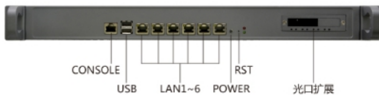
图一：前面板 IO 接口图
