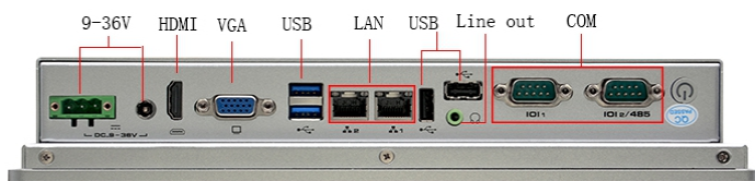
图二：底部 IO 接口图
