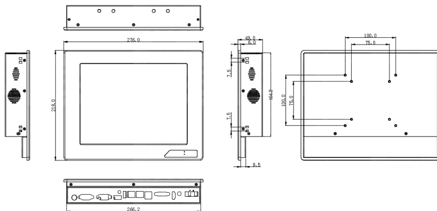
P1021Z-R2 尺寸图
