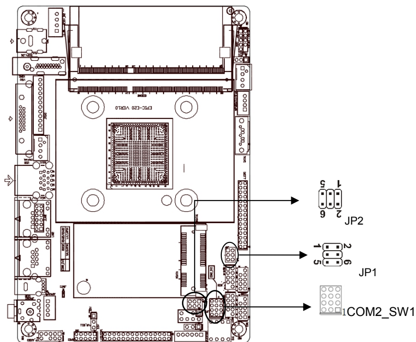
(主板示意图)
