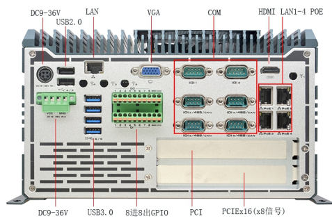
后置IO接口图
