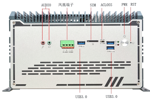
前置IO接口图
