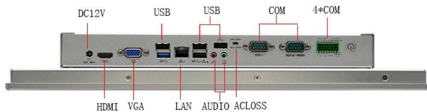
底部I/O视图
