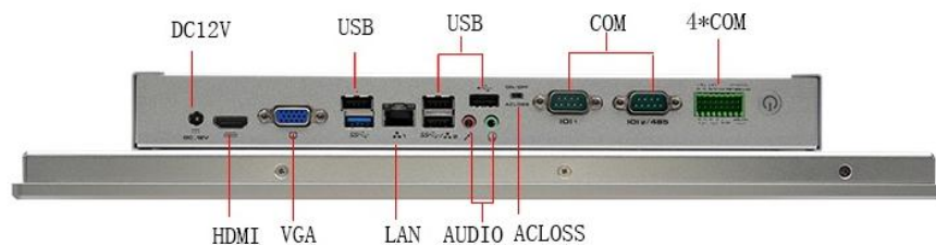
底部I/O视图
