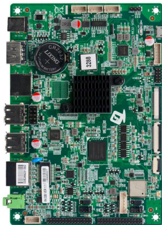
RK32B VER1.1 主板正面图
