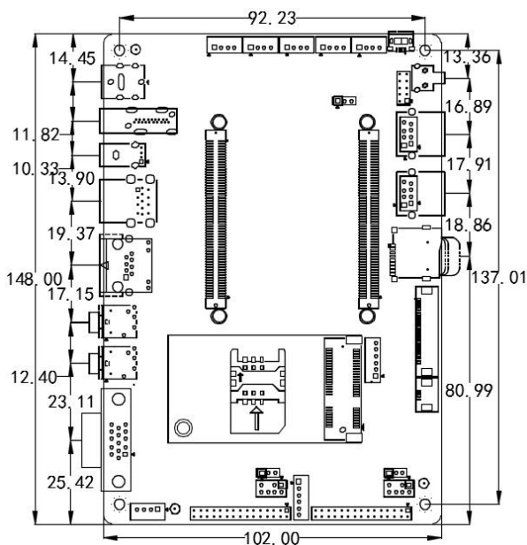
CK33-V 底板尺寸图
