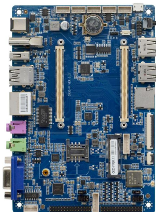
图三：CK33-V 底板正面图
