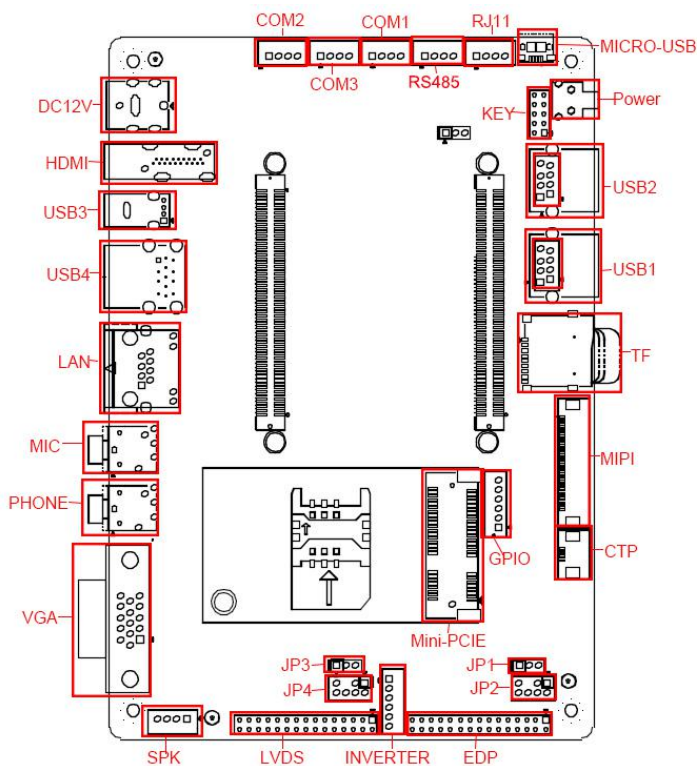
CK33-V 接口示意图
