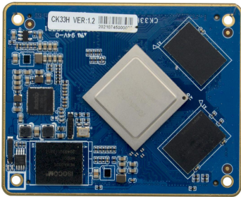
图一： CK33 核心板产品正面图
