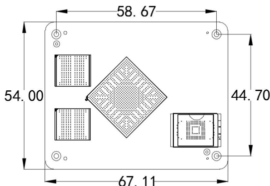
CK33 核心板尺寸图
