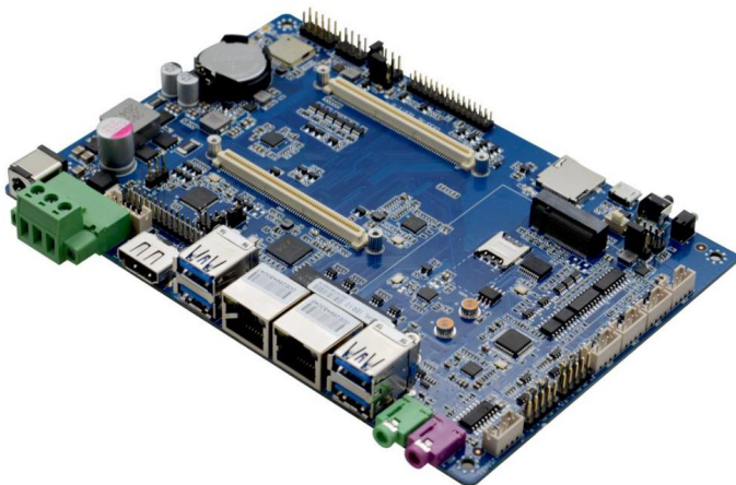
CK33-HL VER1.0 主板正面 IO 图
