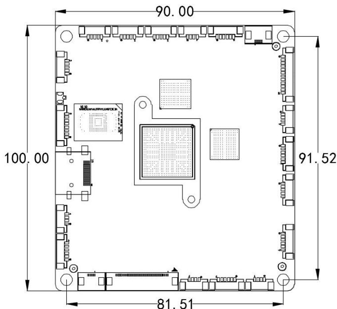
TS32 VER:1.0 主板尺寸图
