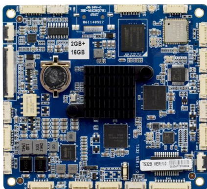
图一：TS32 主板正面图
