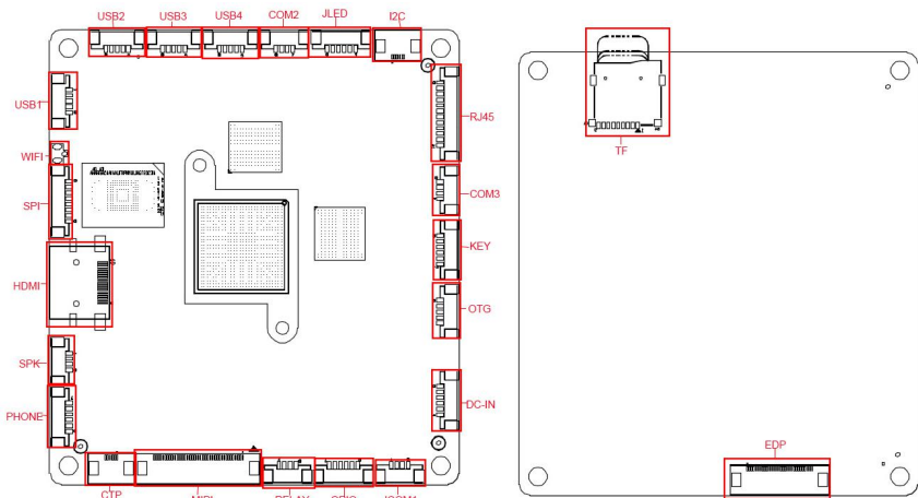
TS32 VER:1.0 接口位置图
