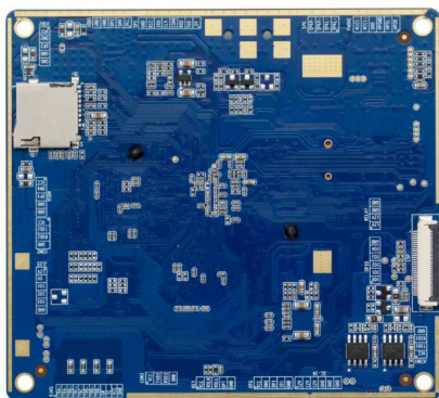
图二：TS32 主板背面图
