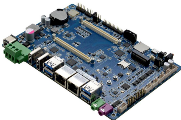
CK33-H2 VER1.0 主板正面 IO 图
