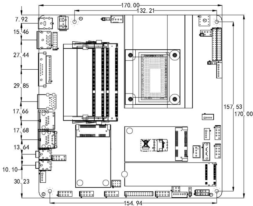
ITX-B672 VER:1.0尺寸图
