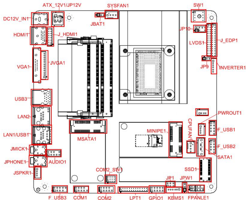
ITX-B672 接口位置图
