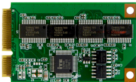
图二： TPM-4COM VER:1.0 产品背面图
