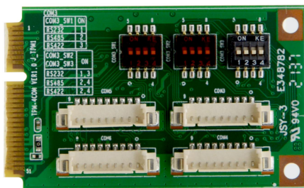
图一： TPM-4COM VER:1.0 产品正面图
