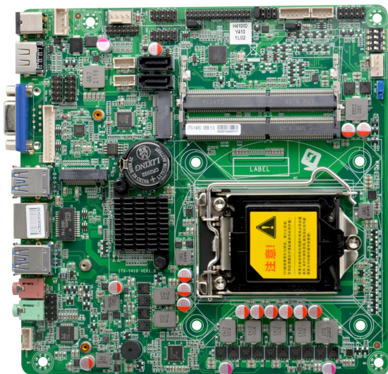
图一：ITX-Y410 VER1.0 正面图
