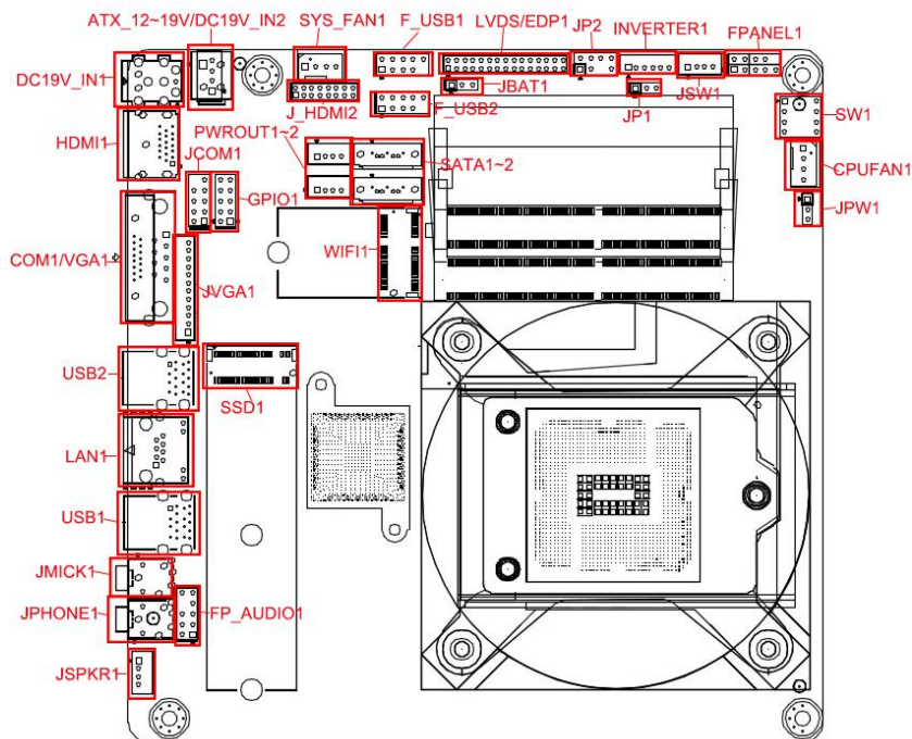
ITX-Y410 VER1.0 接口位置图
