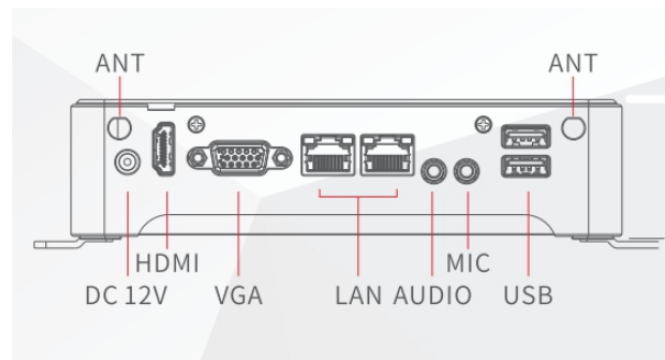
后面板外置I/O视图
