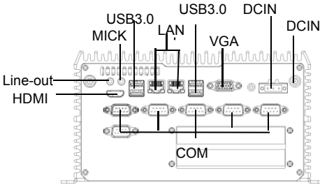
后面板外置I/O视
