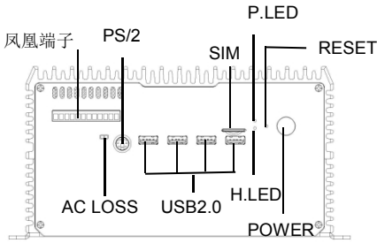
前面板外置I/O视
