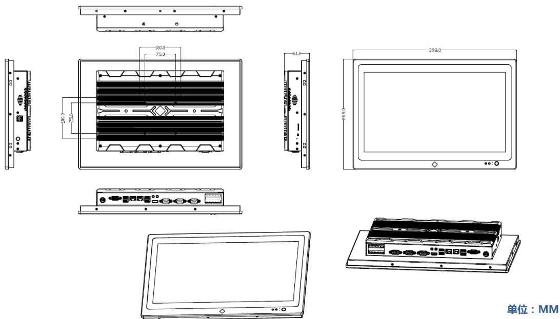
正背面视图
