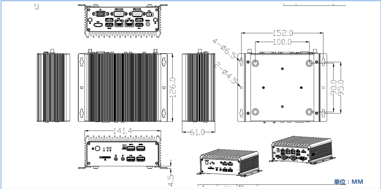
尺寸图
