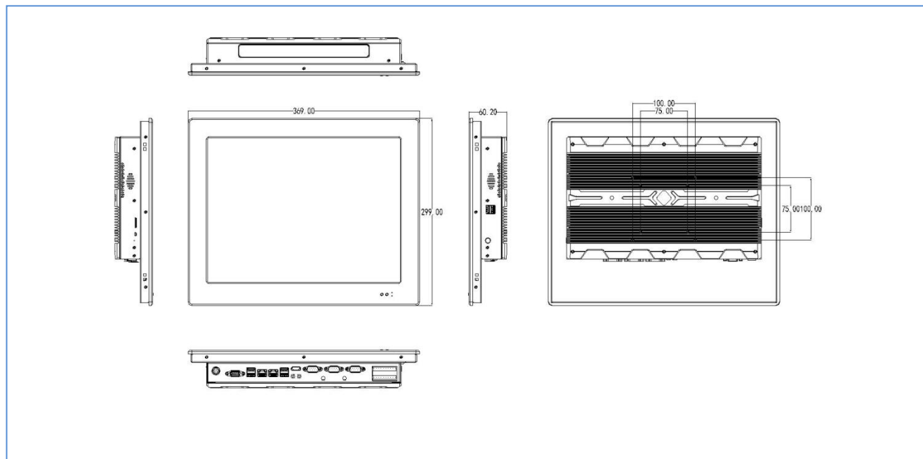
前后面板视图
