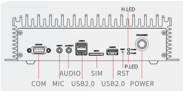
前面板外置I/O视图
