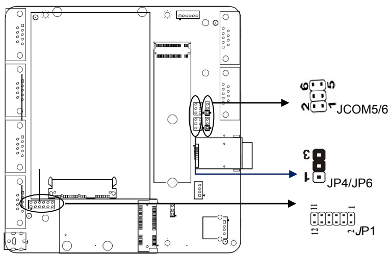
(N81-VGA 示意图)
