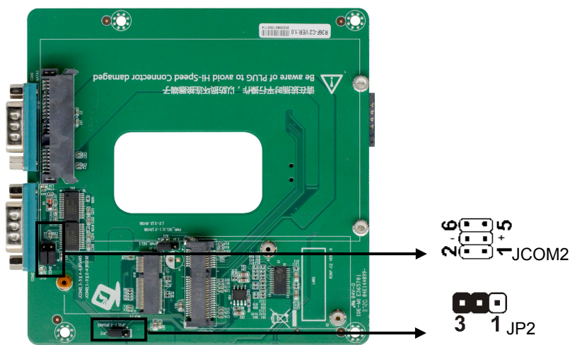
(R36F-C2 IO 板图)
