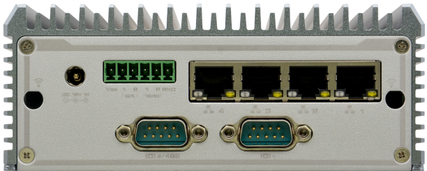
图二：C4350S-L4 后置IO图
