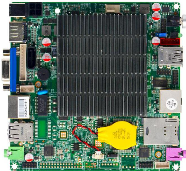
STX-N29 VER:1.6 主板正面图
