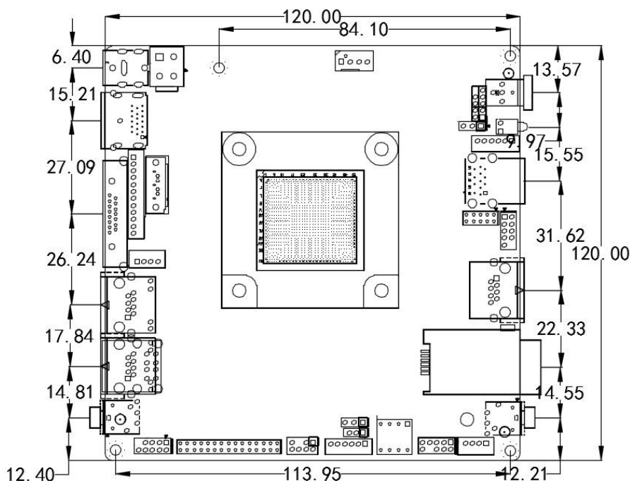
STX-N29 VER:1.6 尺寸图
