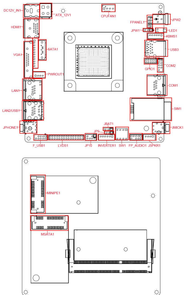
STX-N29 VER:1.6 接口示意图
